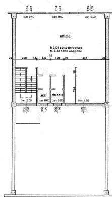
Pianta piano primo
