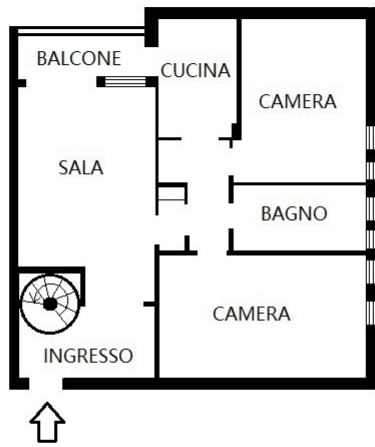
PIANTA PIANO QUARTO
