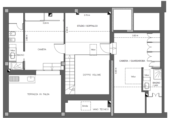
PIANTA SOTTOTETTO
